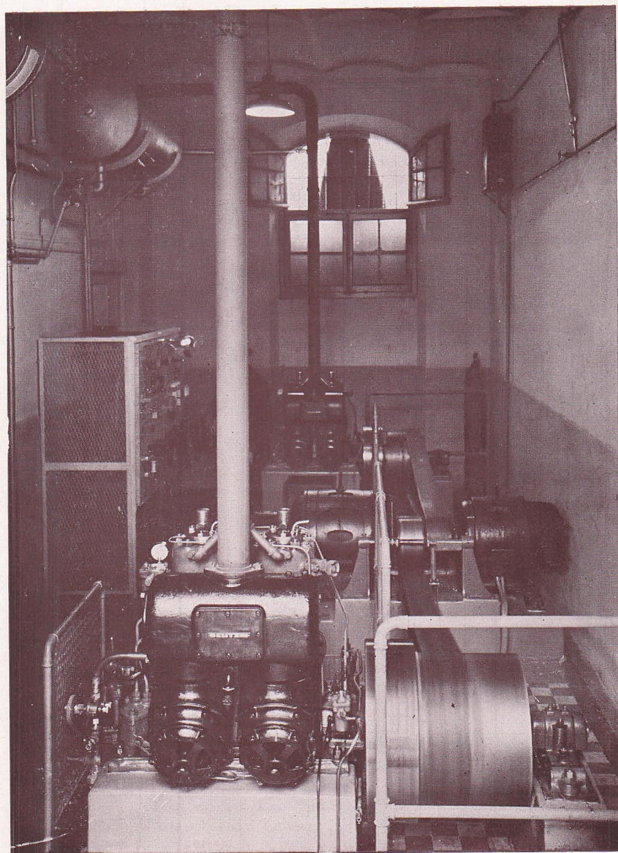
LA CENTRALE ELECTRIQUE. Deux moteurs Diesel-Deutz verticaux actionnent deux groupes électrogènes : l'un avec génératrice à courant continu pour la lumière, l'autre avec un alternateur triphasé pour la force motrice.
